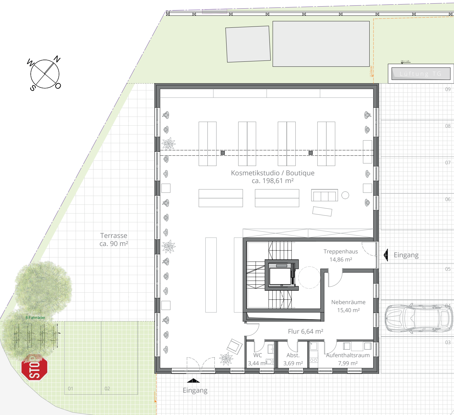
Erdgeschoss | Haus M
